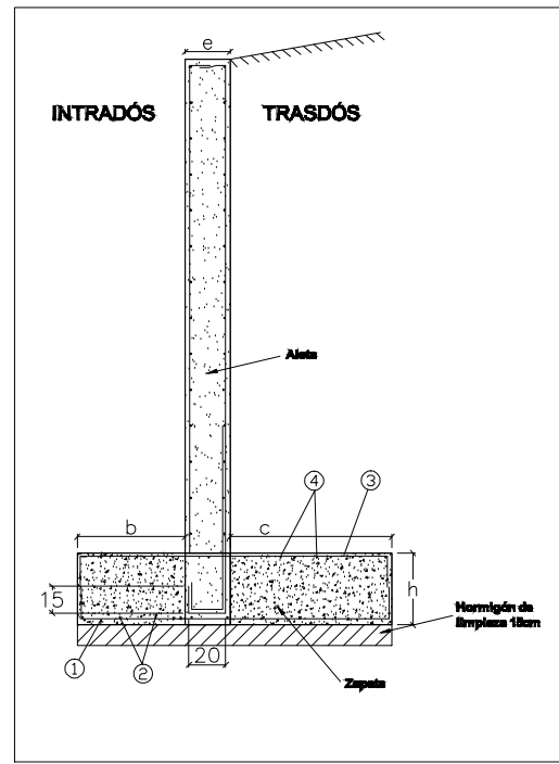
Armado de la zapata de la aleta H1 T1
