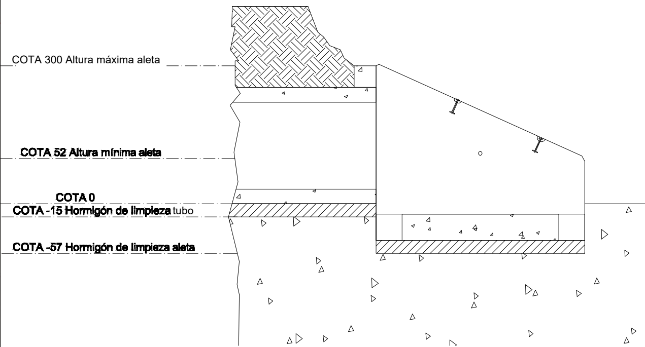
UNIÓN DE ALETA CON EL TUBO
