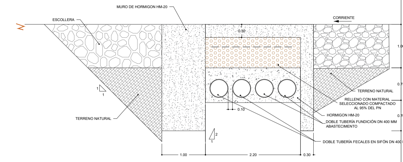
PROTECCION EN CRUCE DE RIO O VAGUADA
