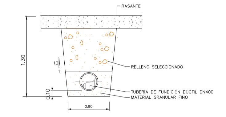
SECCION TIPO DE ZANJA EN ACERA
