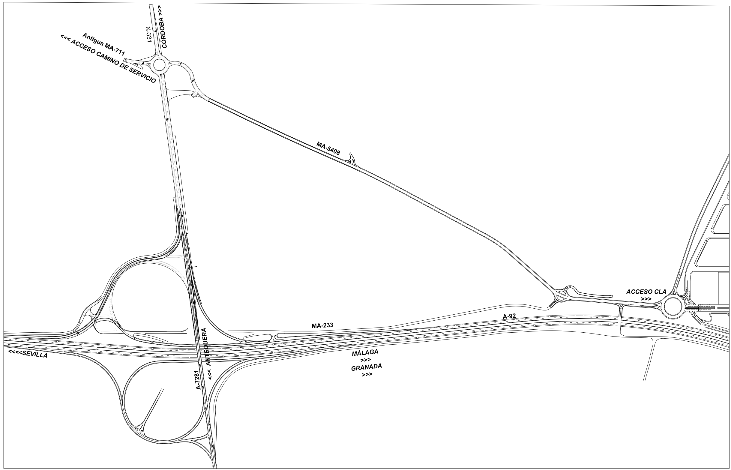
MEJORA DE LA CARRETERA MA-5408 Y ACCESOS A CENTRO LOGÍSTICO DE ANTEQUERA
