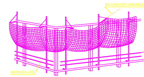
REDES PERIMETRALES CON SOPORTE METALICO TIPO HORCA
