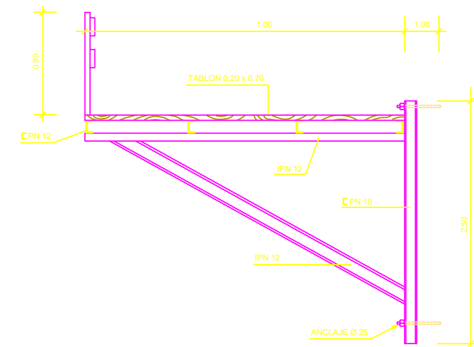
PLATAFORMA DE TRABAJO
