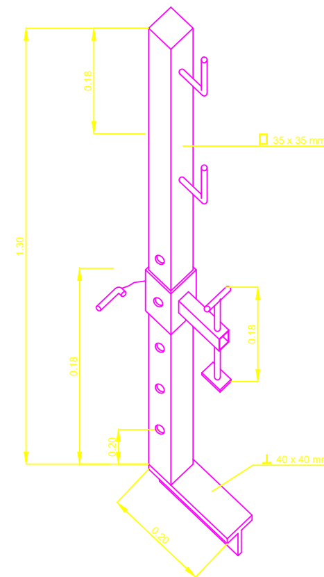
BARANDILLAS TIPO SARGENTO: CON BARANDILLA METALICA.
